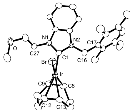
Figure 1. Molecular structure of complex 1a (hydrogen atoms have been omitted). Selected bond lengths [Å] and angles [°]: \text{Ir}-\text{Br} 2.4920(6), \text{Ir}-\text{C1} 2.008(4), \text{Ir}-\text{C8} 2.103(5), \text{Ir}-\text{C9} 2.114(5), \text{Ir}-\text{C12} 2.213(5), \text{Ir}-\text{C13} 2.193(4), \text{N1}-\text{C1} 1.351(5), \text{N2}-\text{C1} 1.362(6), \text{C8}-\text{C9} 1.392(7), \text{C12}-\text{C13} 1.396(7); \text{Br}-\text{Ir}-\text{C1} , 87.81(12), \text{Br}-\text{Ir}-\text{C8} 162.54(14), \text{Br}-\text{Ir}-\text{C9} 158.9(2), \text{Br}-\text{Ir}-\text{C12} 93.63(14), \text{Br}-\text{Ir}-\text{C13} 91.46(13), \text{C1}-\text{Ir}-\text{C8} 93.1(2), \text{C1}-\text{Ir}-\text{C9} 92.4(2), \text{C1}-\text{Ir}-\text{C12} 163.4(2), \text{C1}-\text{Ir}-\text{C13} 159.7(2), \text{C8}-\text{Ir}-\text{C9} 38.6(2), \text{C8}-\text{Ir}-\text{C12} 90.4(2), \text{C8}-\text{Ir}-\text{C13} 81.6(2), \text{C9}-\text{Ir}-\text{C12} 80.4(2), \text{C9}-\text{Ir}-\text{C13} 95.5(2), \text{C12}-\text{Ir}-\text{C13} 36.9(2), \text{N1}-\text{C1}-\text{N2} 106.4(4).
